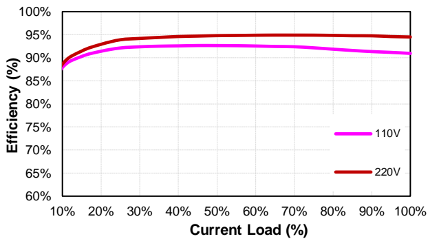
LFM200M300 (Eff Vs Io)
