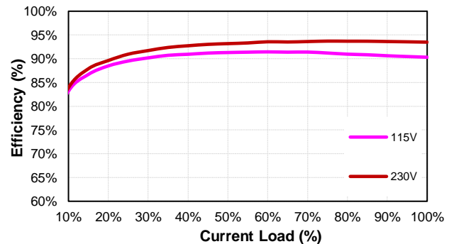
LFM200M150 (Eff Vs Io)
